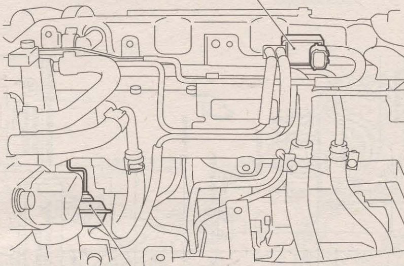
Вакуумный исполнительный элемент клапана завихрения
